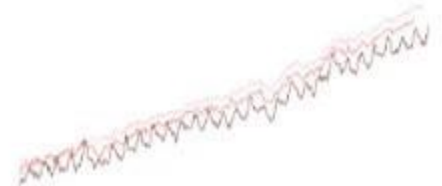
Nivel de océanos
