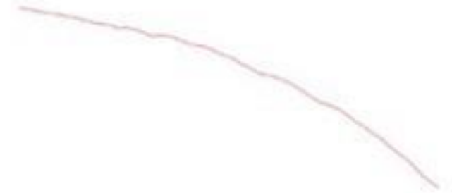
Masa de los glaciares
